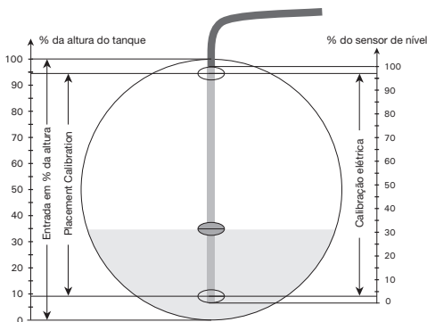
Figura 1 , a seção transversal do tanque cilíndrico horizontal
